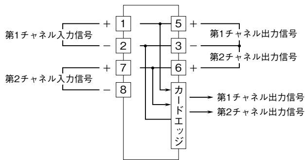
端子接続図
