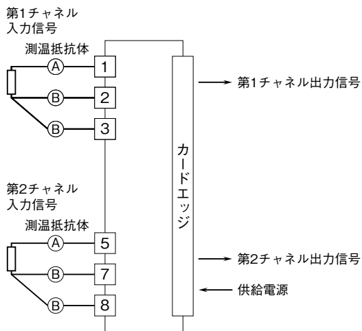
端子接続図
