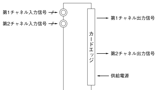
端子接続図
