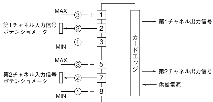
端子接続図
