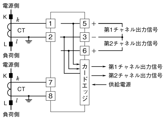
端子接続図
