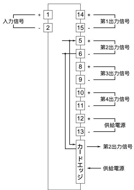
端子接続図
