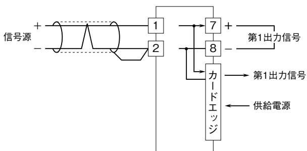
端子接続図
