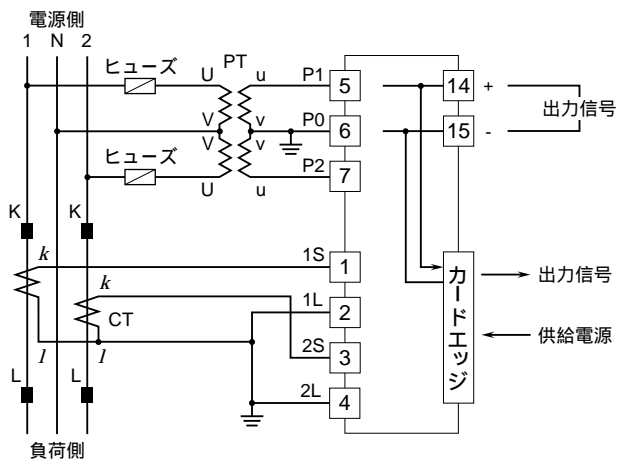
単相3線式
