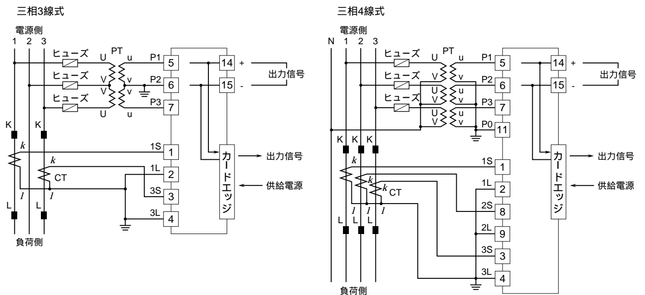
端子接続図
