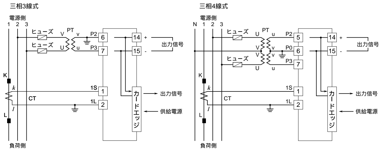
端子接続図
