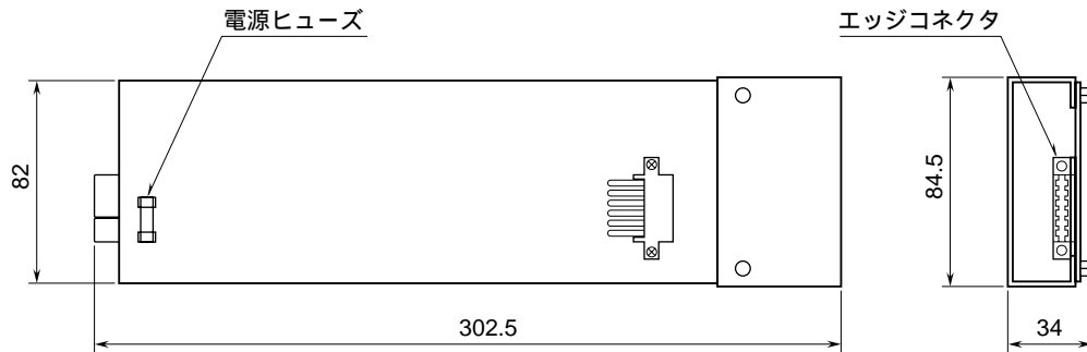
外形寸法図 (単位: mm)
