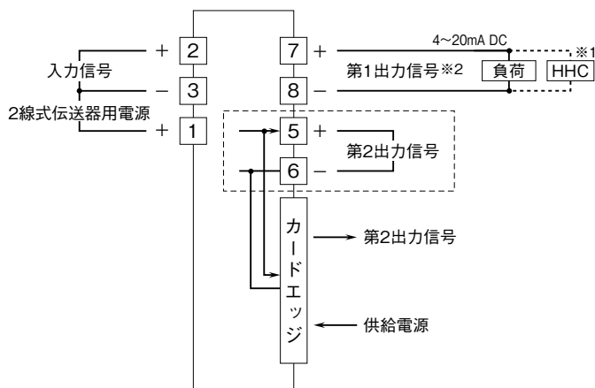
端子接続図
