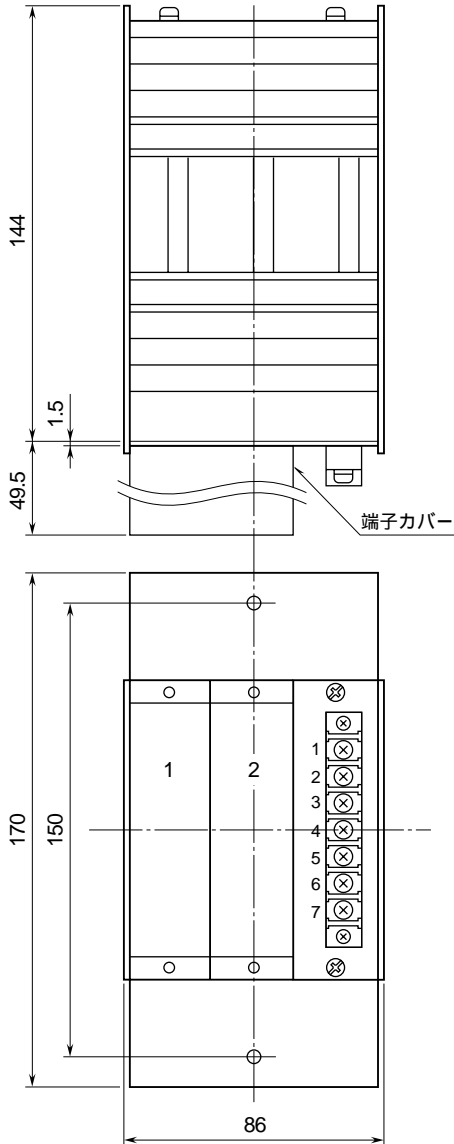
外形寸法図 (単位: mm)
