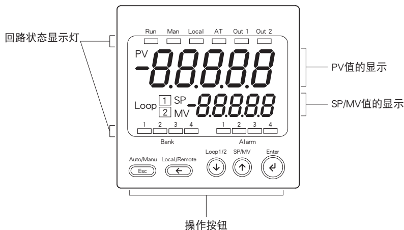
■正面图
