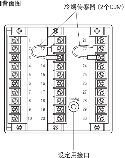
■背面图
