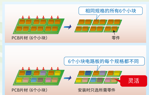
混合PCB贴片生产线
