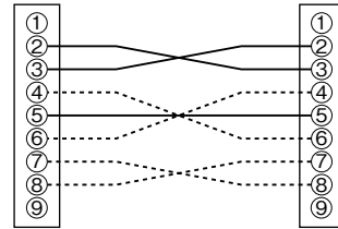
R1MシリーズI/Oなど R2M-2G3
