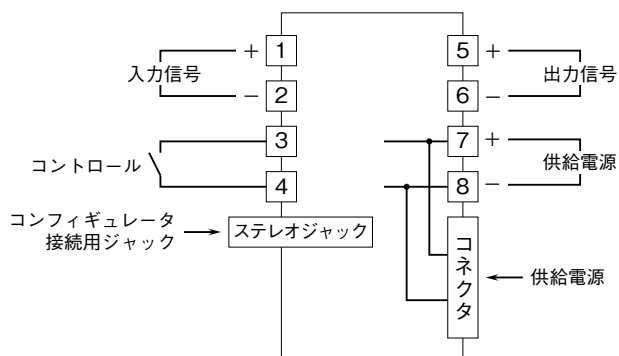
端子接続図
