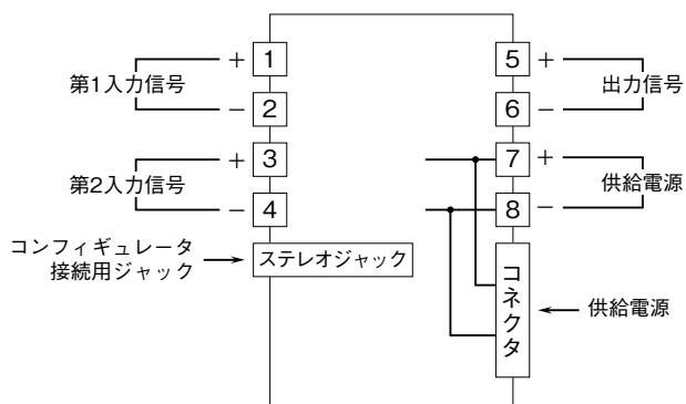
端子接続図
