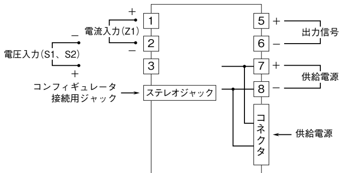
端子接続図
