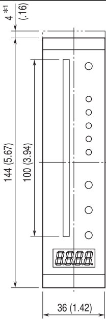
STANDARD BEZEL *2
